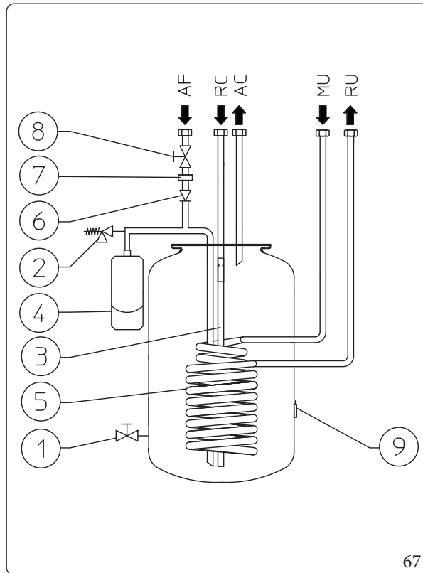
Unità bollitore Inox 80 Litri
