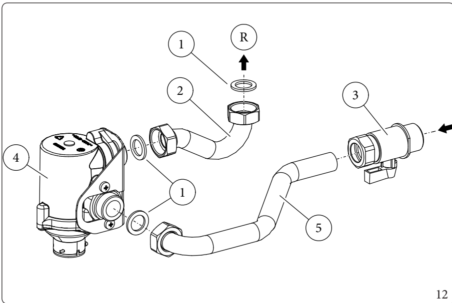
Legenda (Fig. 12): 1 - Guarnizioni piane 2 - Tubo allacciamento ritorno 3 - Rubinetto di intercettazione 4 - Filtro cicloidale 5 - Tubo allacciamento mandata impianto
