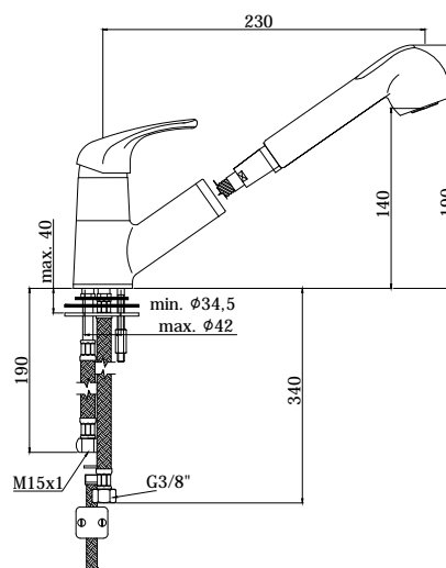
DISEGNO TECNICO
