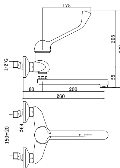
DISEGNO TECNICO
