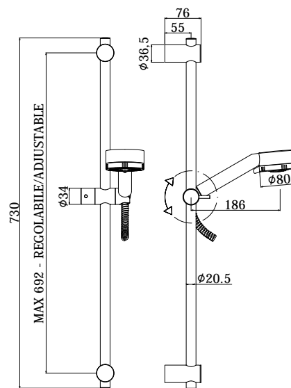
DISEGNO TECNICO
