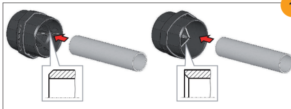
Sbavare il tubo internamente ed esternamente (Fig.1) / Debur pipe inside and outside (Pic.1)
