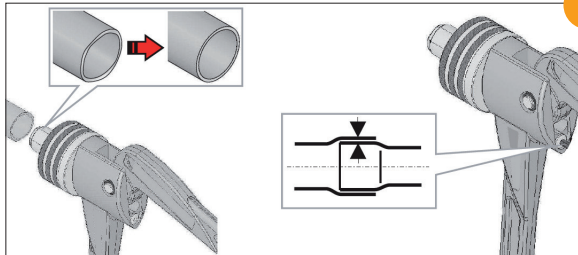
Inserire il tubo fino alla battuta (Fig.2) / Slip on pipe up to the stop (Pic.2)
